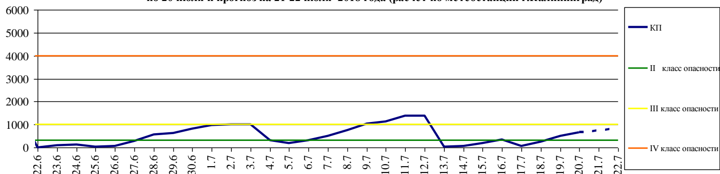
Комплексный показатель пожарной опасности лесов по условиям погоды за период с 22 июня по 20 июля и прогноз на 21-22 июля 2018 года (расчёт по метеостанции г.Калининград)
