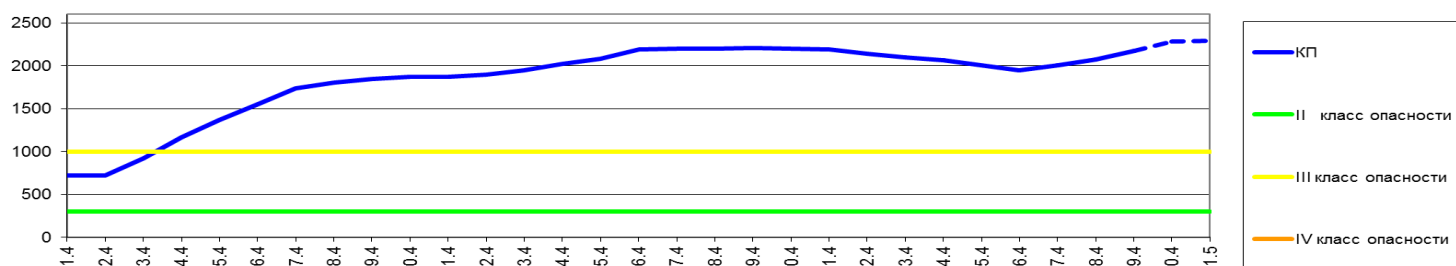
Комплексный показатель пожарной опасности лесов по условиям погоды за период с 01 апреля по 29 апреля и прогноз на 30.04-01.05 2019 года (расчёт по метеостанции г.Калининград)
