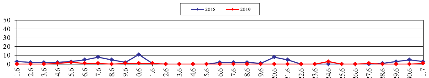
Площадь ландшафтных пожаров, га (2018, 2019 гг., июнь-июль)
