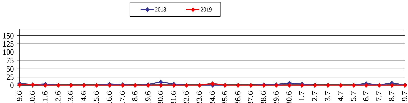
Площадь ландшафтных пожаров, га (2018, 2019 гг., июнь-июль)
