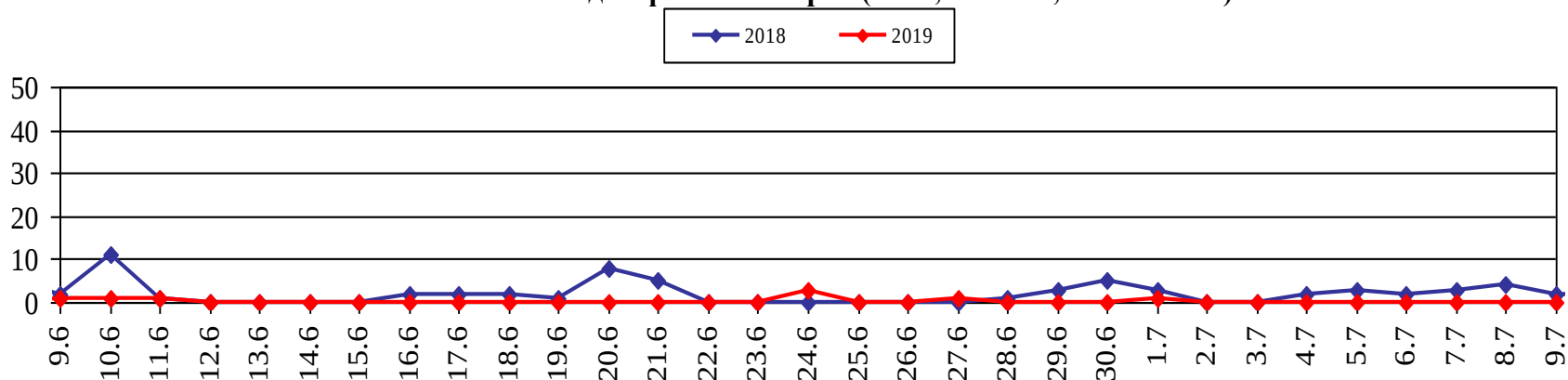
Площадь ландшафтных пожаров, га (2018, 2019 гг., июнь-июль)
