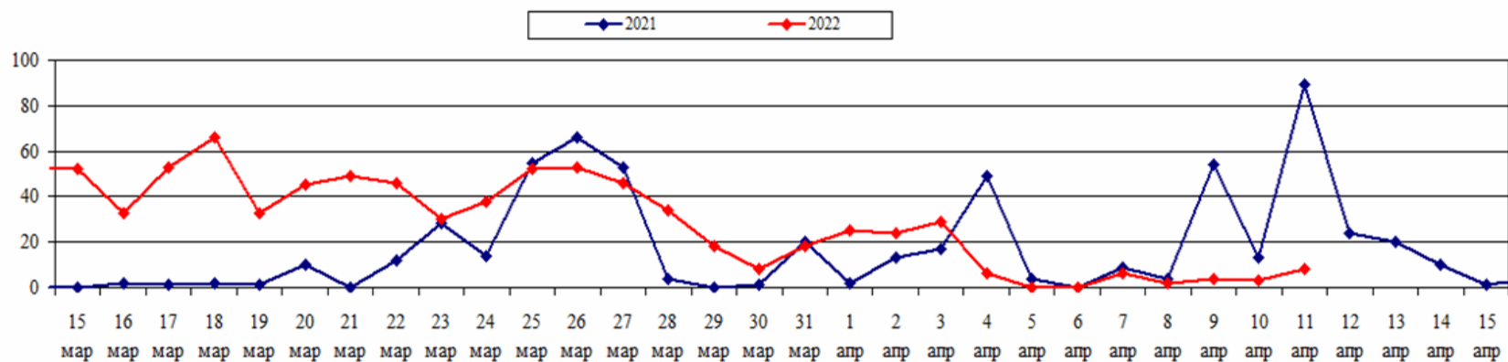
Количество ландшафтных пожаров (2021-2022 гг., март-апрель)
