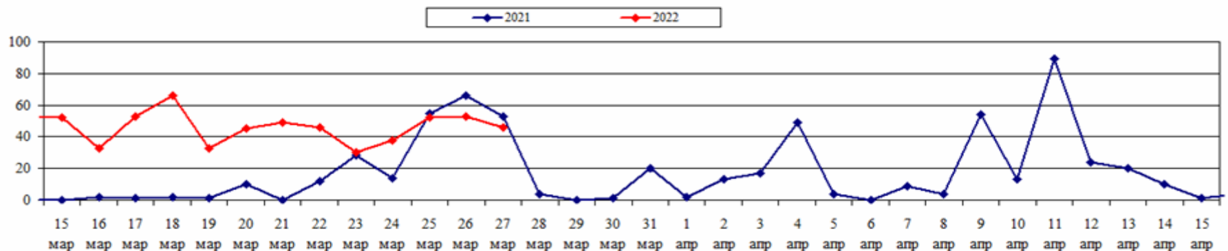
Количество ландшафтных пожаров (2021-2022 гг., март-апрель)
