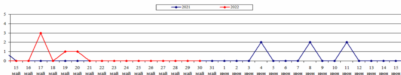
Количество ландшафтных пожаров (2021-2022 гг., май-июнь)
