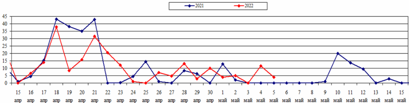
Площадь ландшафтных пожаров (2021-2022 гг., апрель - май)
