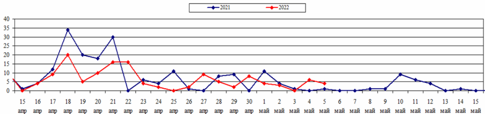
Количество ландшафтных пожаров (2021-2022 гг., апрель - май)
