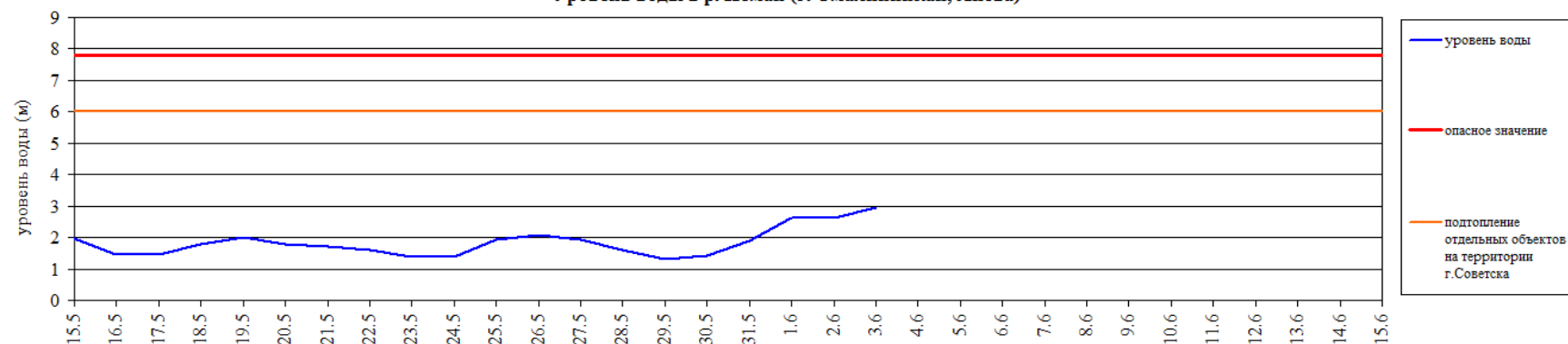
Уровень воды в р. Неман (г. Сматининкай, Литва)
