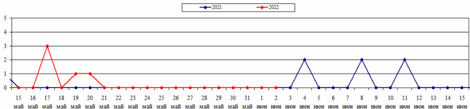
Площадь ландшафтных пожаров (2021-2022 гг., май-июнь)
