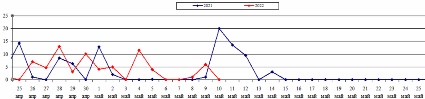
Площадь ландшафтных пожаров (2021-2022 гг., апрель - май)
