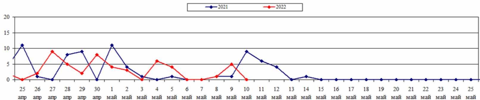
Количество ландшафтных пожаров (2021-2022 гг., апрель - май)
