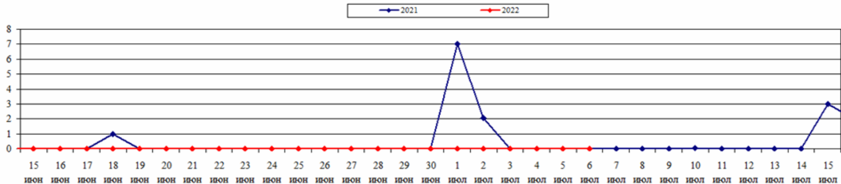
Площадь ландшафтных пожаров (2021-2022 гг., июнь-июль)
