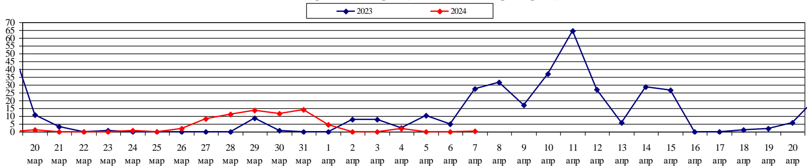
Площадь ландшафтных пожаров (2023-2024 гг. март-апрель)
