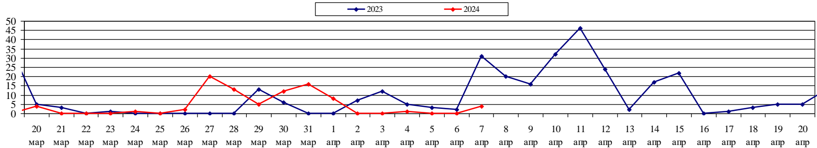
Количество ландшафтных пожаров (2023-2024 гг. март-апрель)
